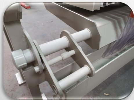
Bandeja pivotante
